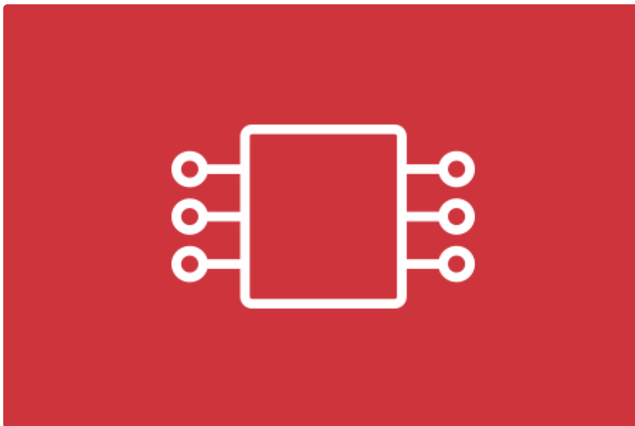
Informatik
